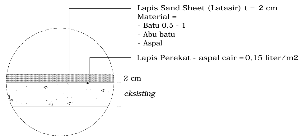
DETAIL PERKERASAN A skala 1 : 10
