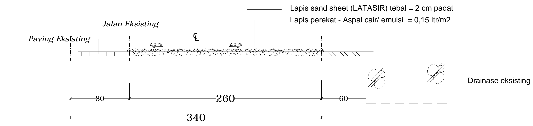
TYPIKAL POTONGAN MELINTANG TYPE-01 ( STA 0+000 - 0+889,72 ) SKALA 1 : 25
